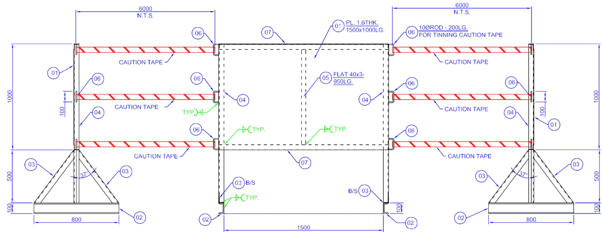
ELEVATION B-B
