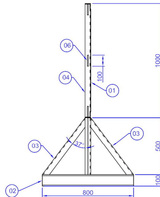
ELEVATION B-B
