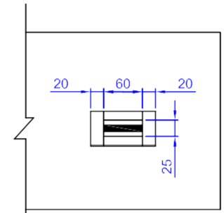
DETAIL - Y SCALE 1:8
