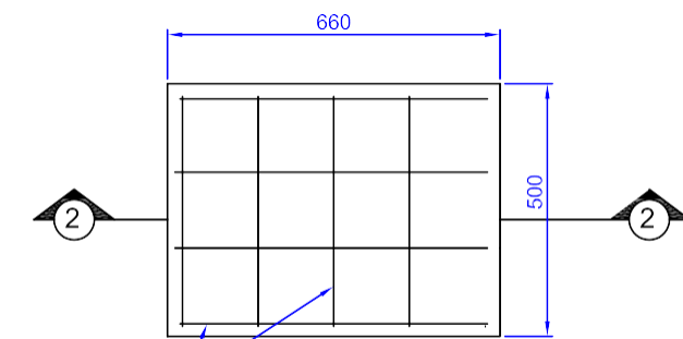
PRECAST RCC SLAB
