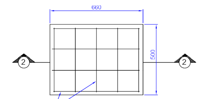
PRECAST RCC SLAB
