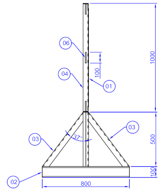
ELEVATION B-B
