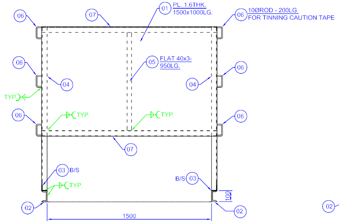
ELEVATION A-A
