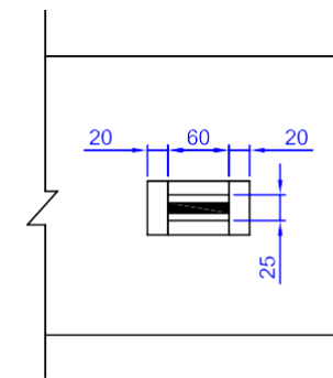
DETAIL - Y SCALE 1:8
